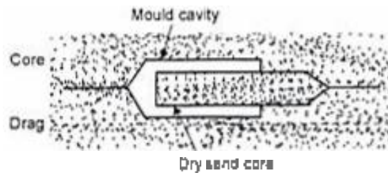
c) Horizontal core
