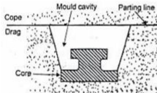
e) Ram-up core
