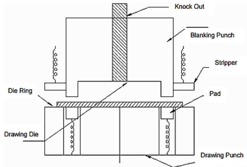
Combination die
