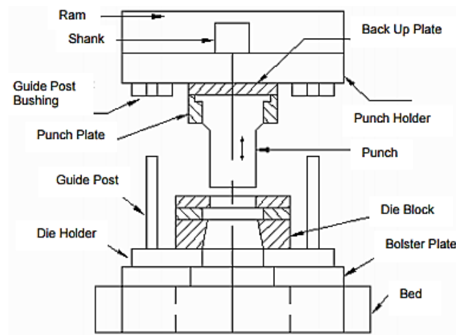
Simple Die
