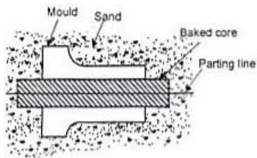
a) Horizontal core
