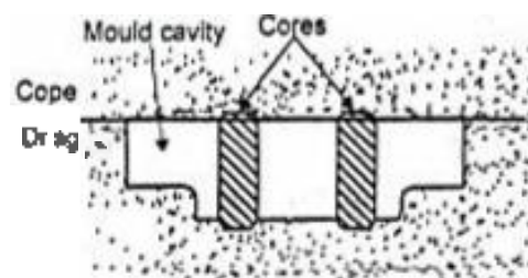
g) Kiss core
