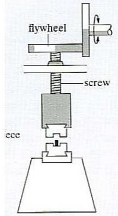
Fig. 3.13 Screw Press
