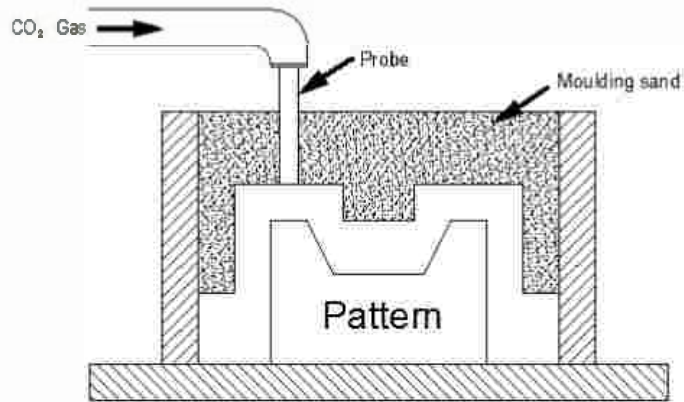
Fig. 1.47 Carbon - di -Oxide Processes
